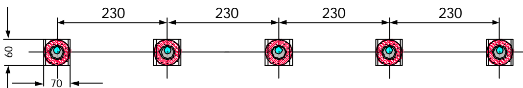
Anordnung der Fundamentaussparungen bei einer 4-fachen Versenkrechanlage:
